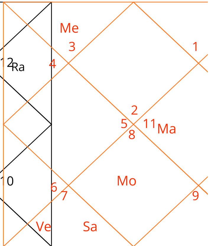
Trimsamsa (D-30)
