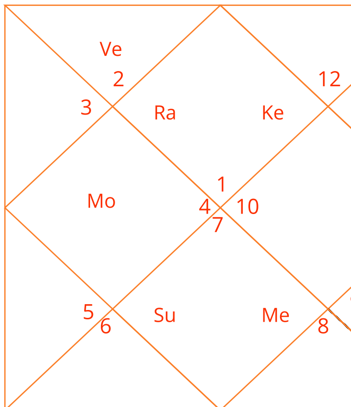
Khavedamsa (D-40)
