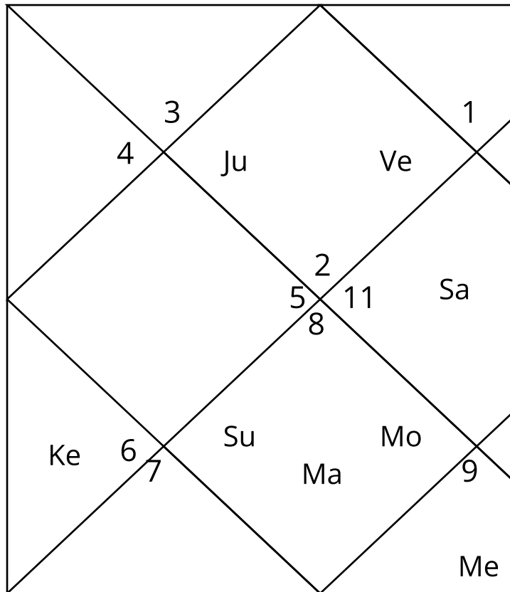
Saptavimsamsa
